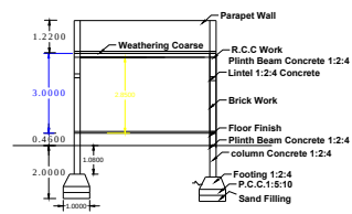
SECTION - AB
