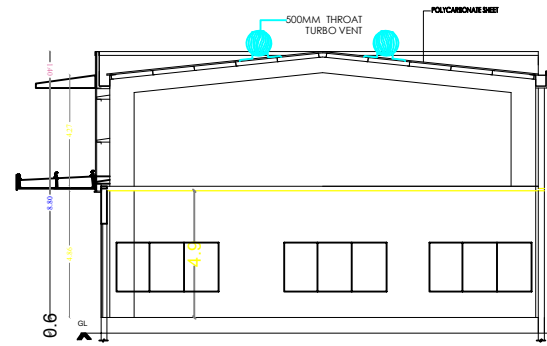
SECTION A-B
