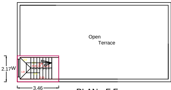
PLAN - F.F.
