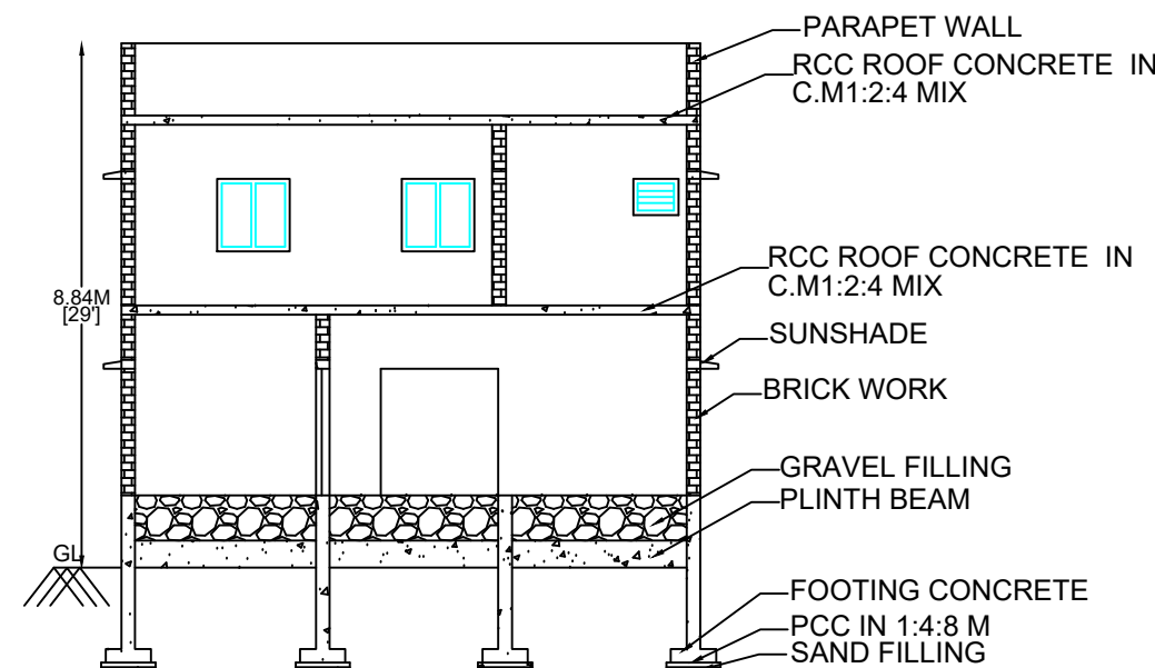
SECTION A-B
