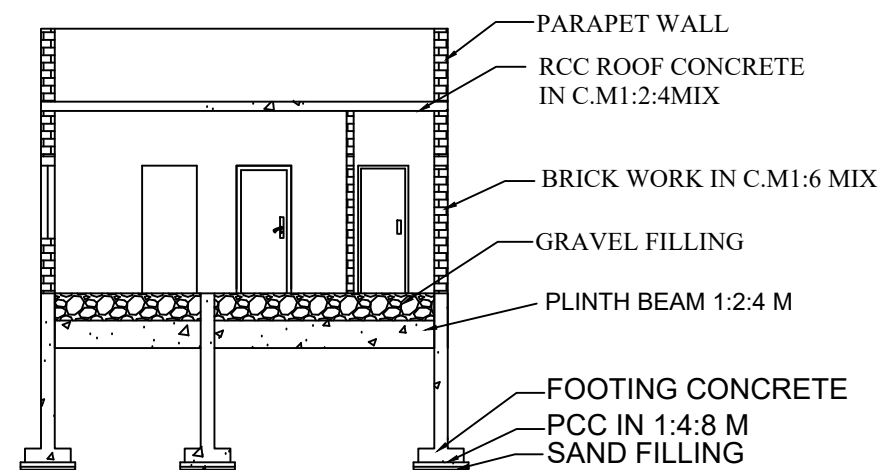
SECTION A-B
