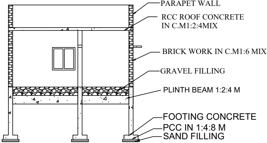
SECTION A-B
