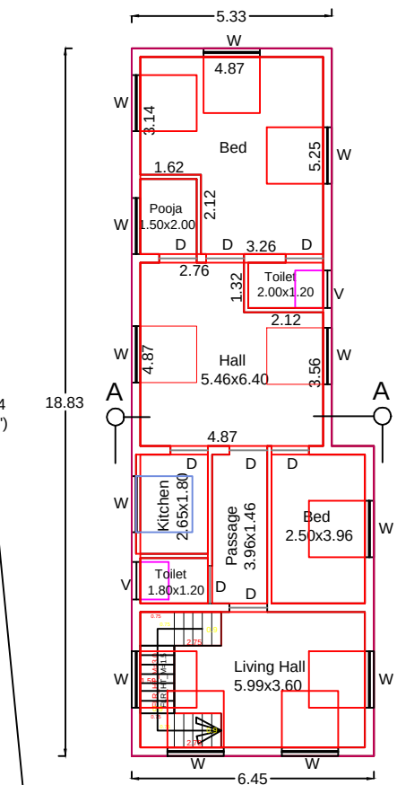
PLAN - F.F
