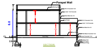
SECTION - AB
