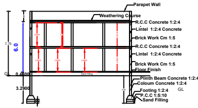
SECTION - AB
