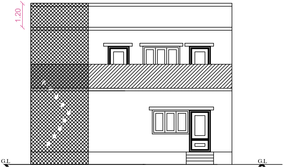
ELEVATION
