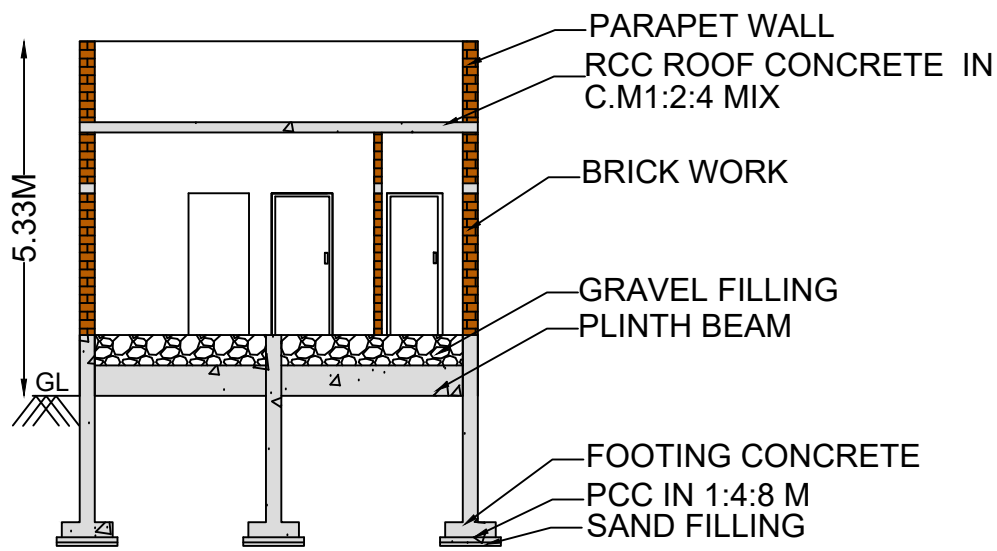
SECTION A-B
