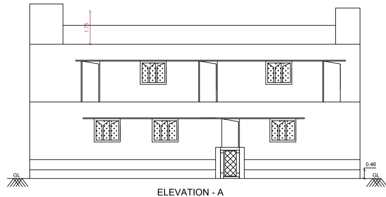
ELEVATION - A
