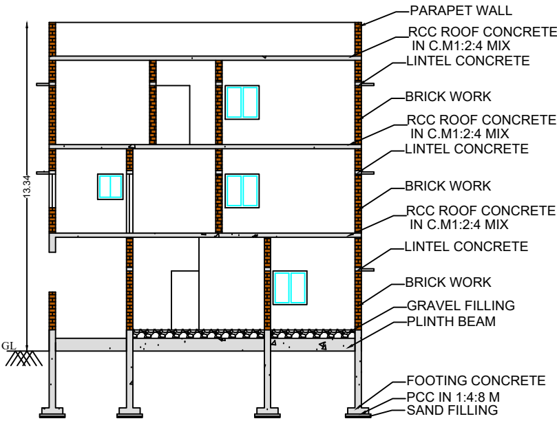
SECTION A-B
