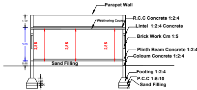
SECTION - AB
