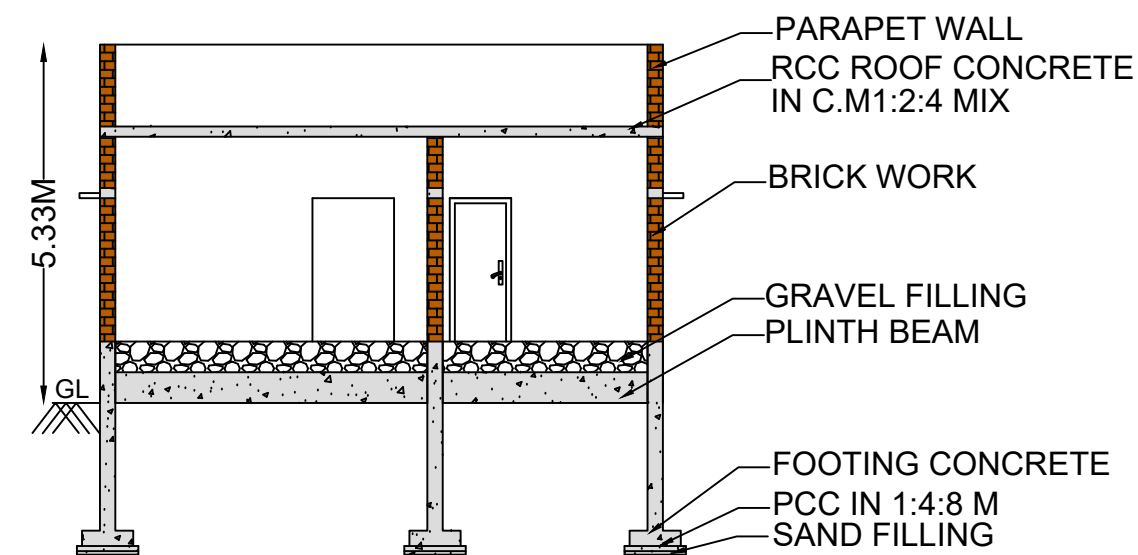
SECTION A-B
