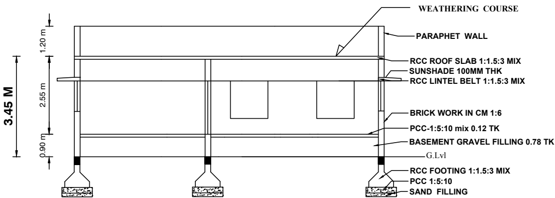
SECTION A-A
