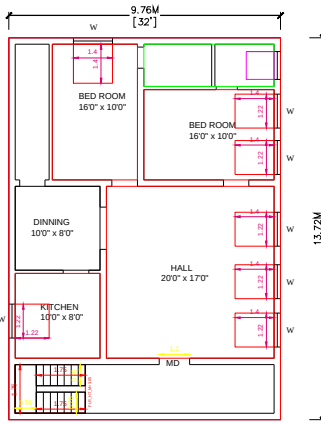
OOR PLAN
