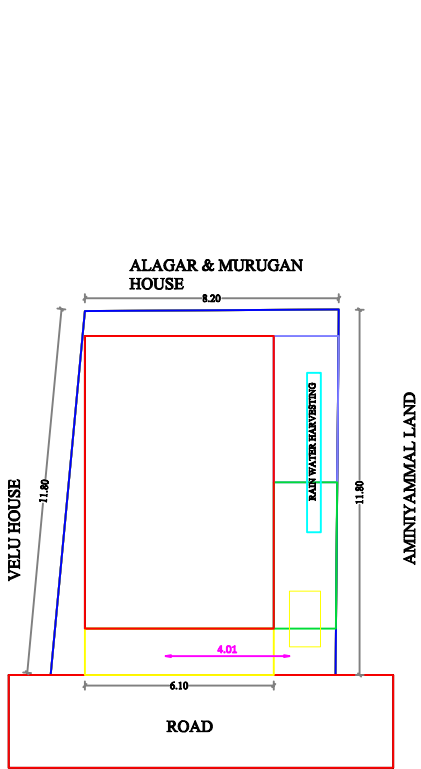
SITE PLAN 1:100
