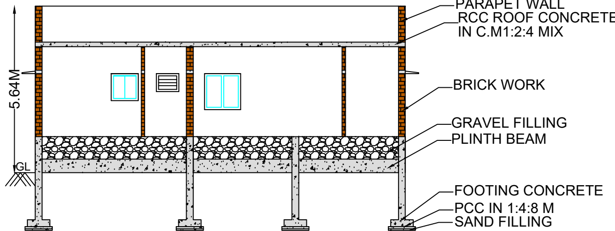
SECTION A-B
