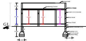
SECTION - AB
