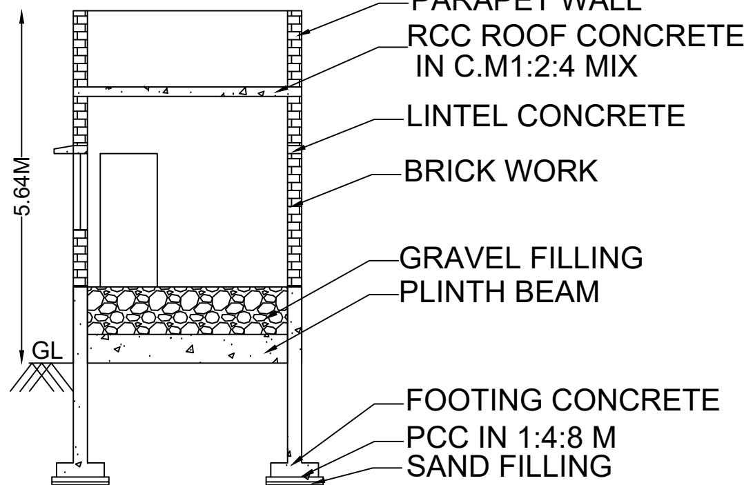
SECTION A-B
