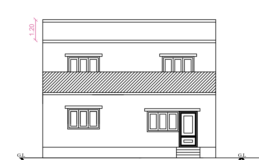
ELEVATION
