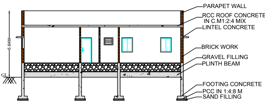
SECTION A-B
