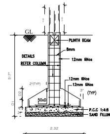
SCALE : 1:50.
