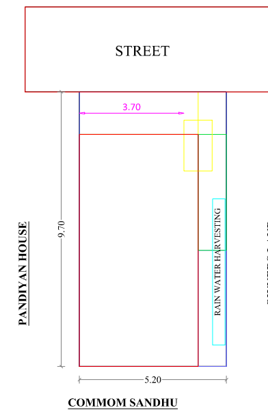
SITE PLAN 1:100
