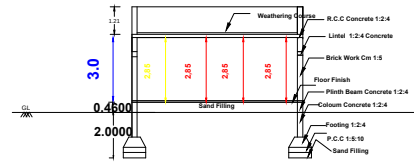
SECTION - AB
