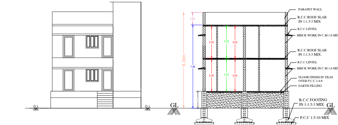
ELEVATION
