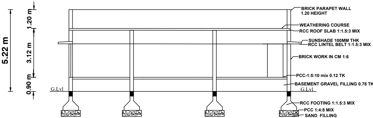
SECTION A-A
