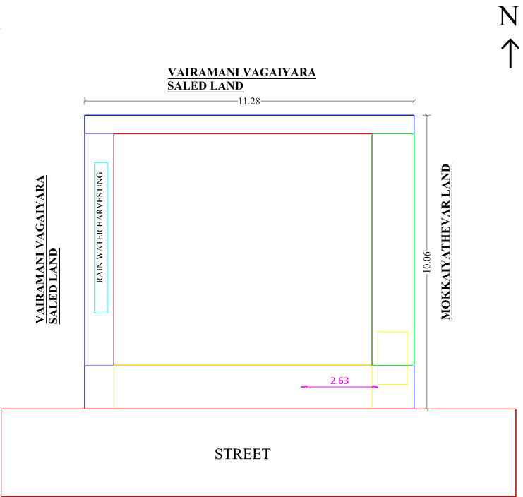
SITE PLAN 1:100
