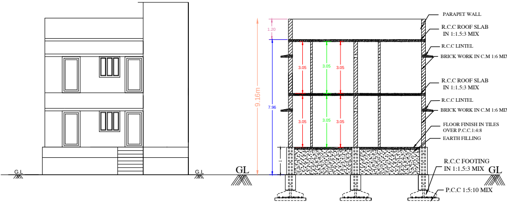
ELEVATION
