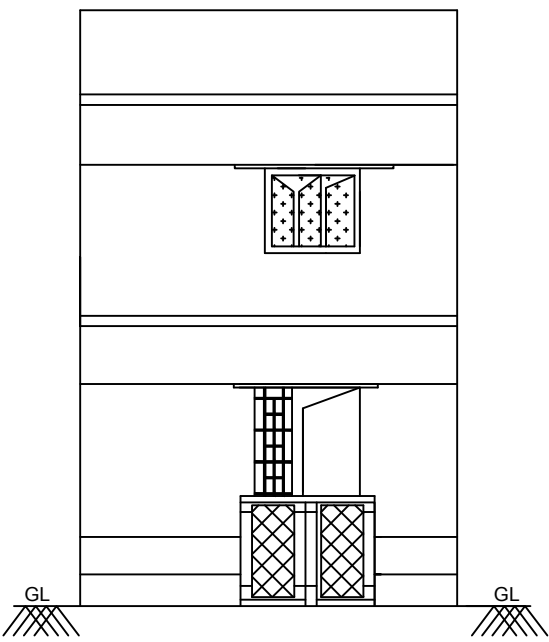
ELEVATION - A
