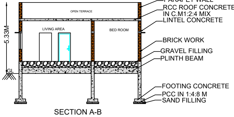
SECTION A-B
