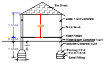
SECTION - AB
