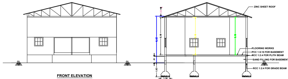
SECTION A-A
