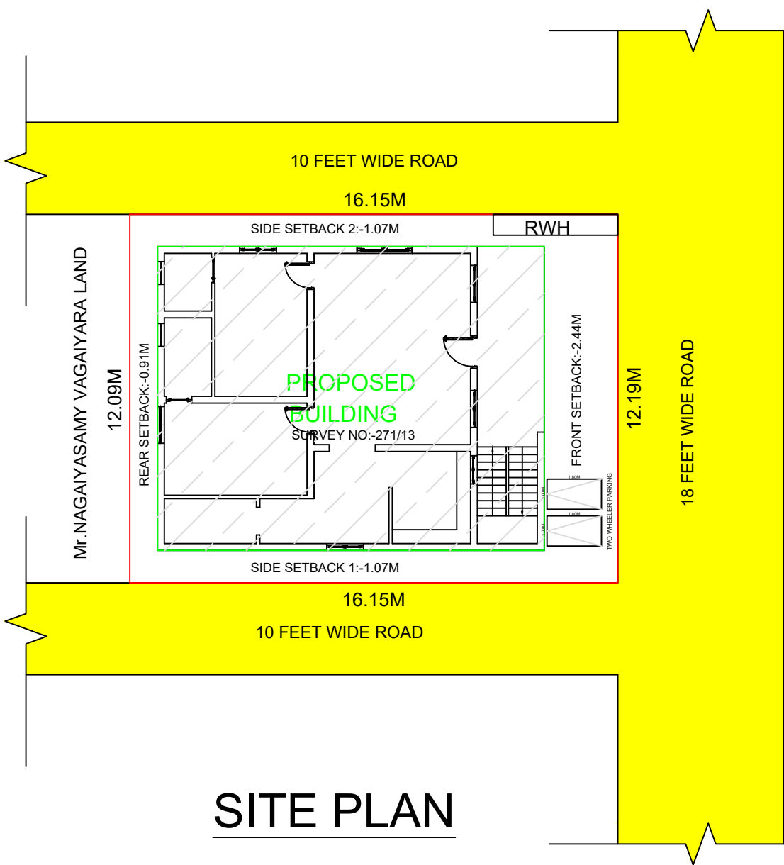
N SITE PLAN SCALE : 1:100
