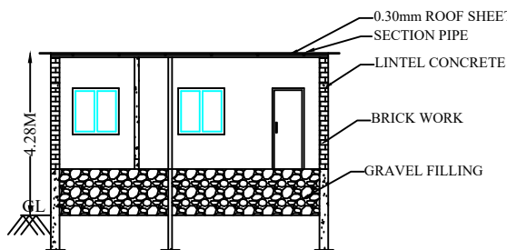
SECTION A-B
