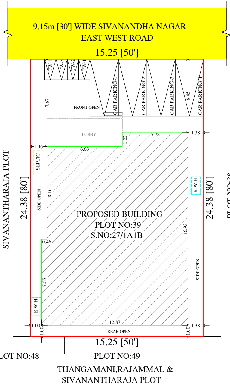
SITE PLAN:
