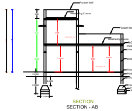
SECTION - AB
