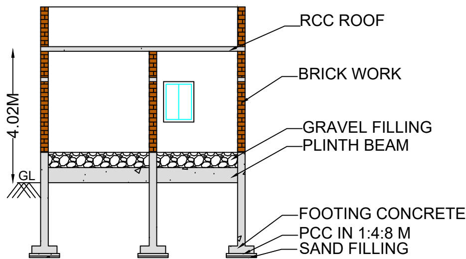
SECTION A-B
