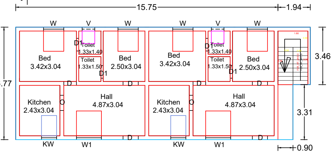
PLAN - G.F
