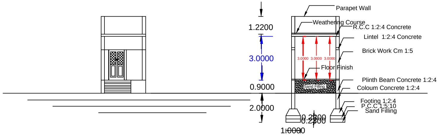
Elevation
