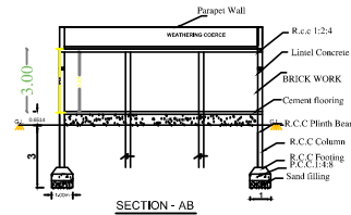
SECTION - AB
