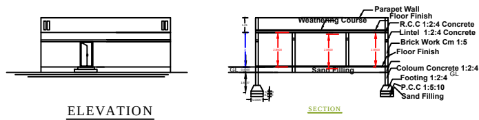
SECTION - AB
