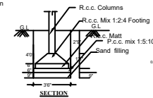
R.C.C. COLUMNS DETAILS
