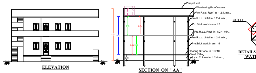
(SCALE - 1:100)
