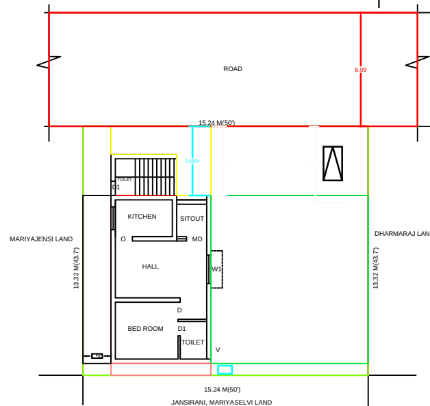
SITE PLAN 1:100
