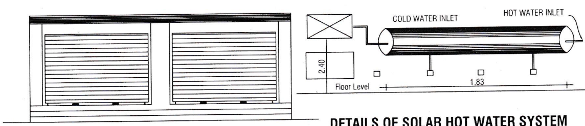
ELEVATION
