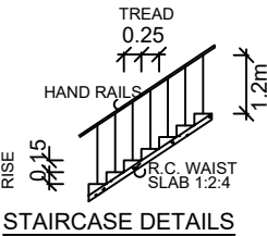
SCALE:- 1:20
