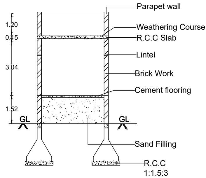
SECTION ON'AB'
