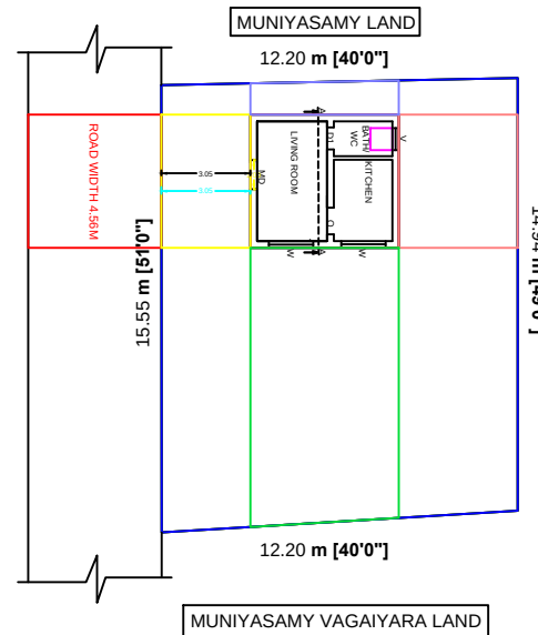
SITE PLAN 1:100
